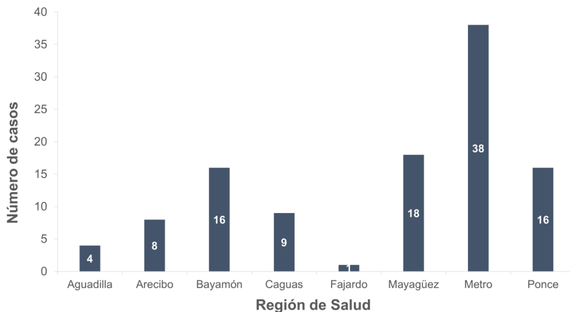
Gráfica 3. Distribución de incidencia acumulada de Enfermedades Transmisibles por Alimentos y/o Agua por región de salud, semana epidemiológica 16, 2023 (N=110)
