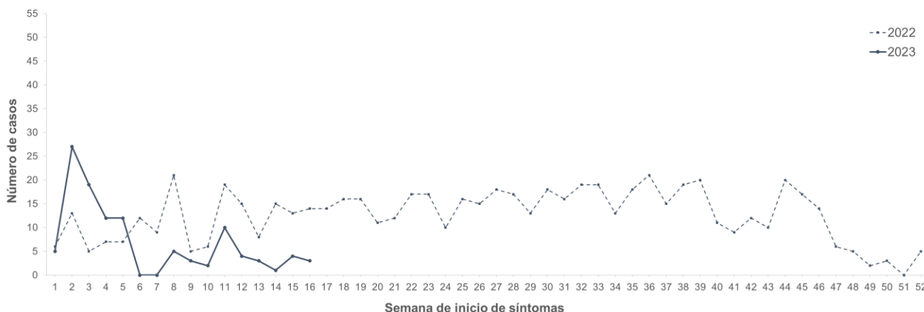
Gráfica 1. Incidencia acumulada de Enfermedades Transmisibles por Alimentos y/o Agua por semana epidemiológica, semana epidemiológica 16, 2023 (N=110)
