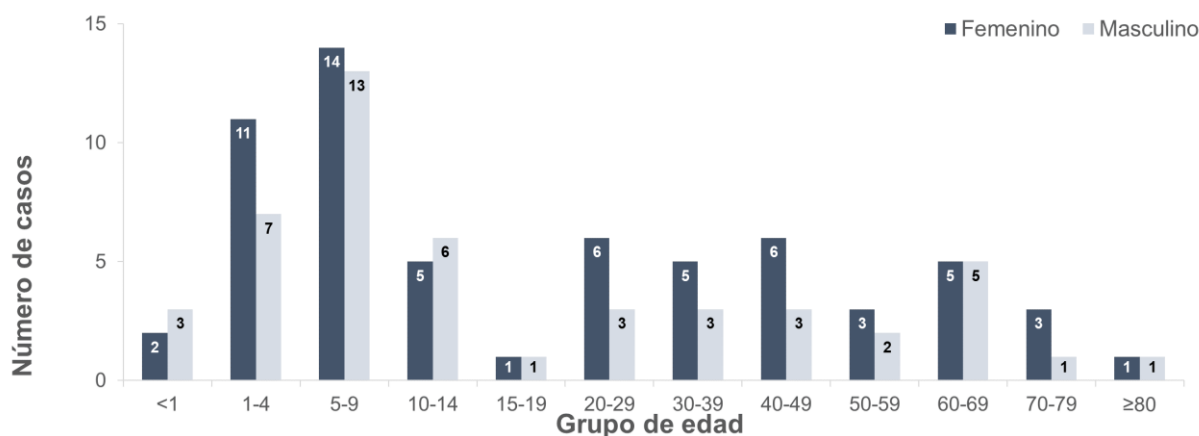
Gráfica 2. Incidencia acumulada de Enfermedades Transmisibles por Alimentos y/o Agua por sexo y grupo de edad, semana epidemiológica 16, 2023 (N=110)
