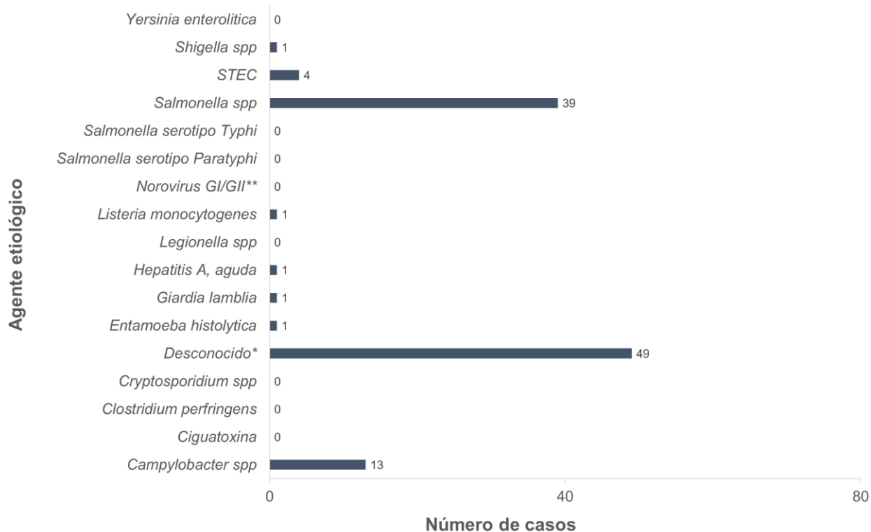
Gráfica 4. Incidencia acumulada de Enfermedades Transmisibles por Alimentos y/o Agua según el agente etiológico, semana epidemiológica 16, 2023 (N=110)
